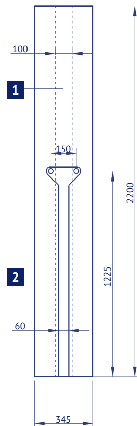
Achterkant van het afgerond bevestigingspaneel (Art. 932.009.0007)
